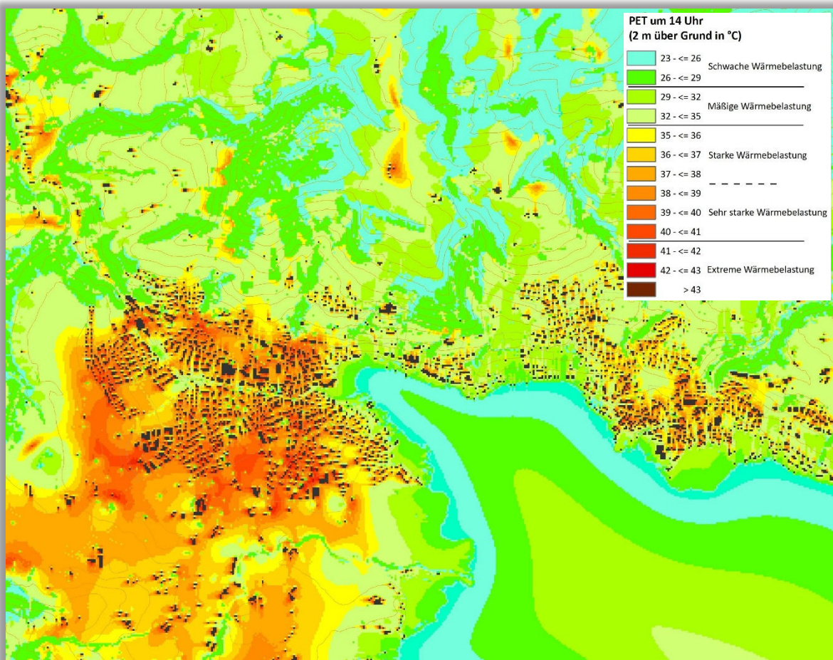
Abb. 4.4: PET im Bereich in Unterägeri und Oberägeri zum Zeitpunkt 14 Uhr mittags (2m ü. Grund)
