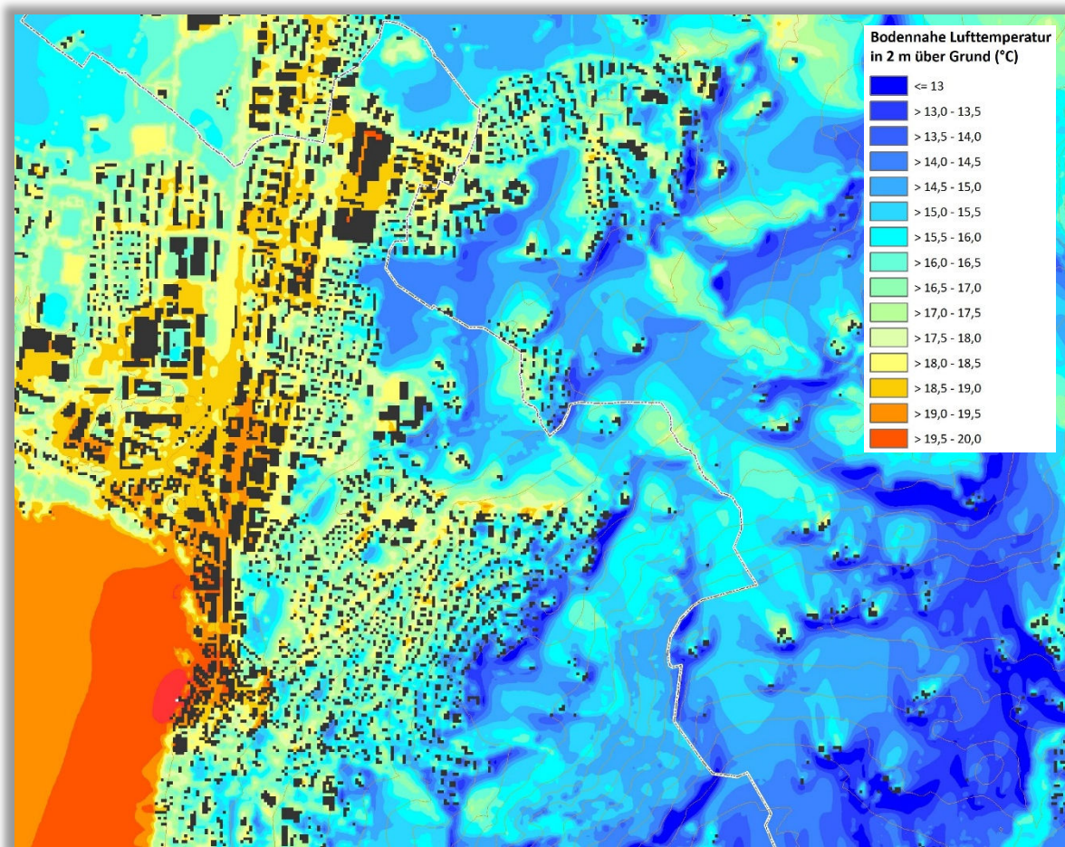
Abb. 4.1: Temperaturfeld in der Stadt Zug zum Zeitpunkt 4 Uhr morgens (2m ü. Grund)
