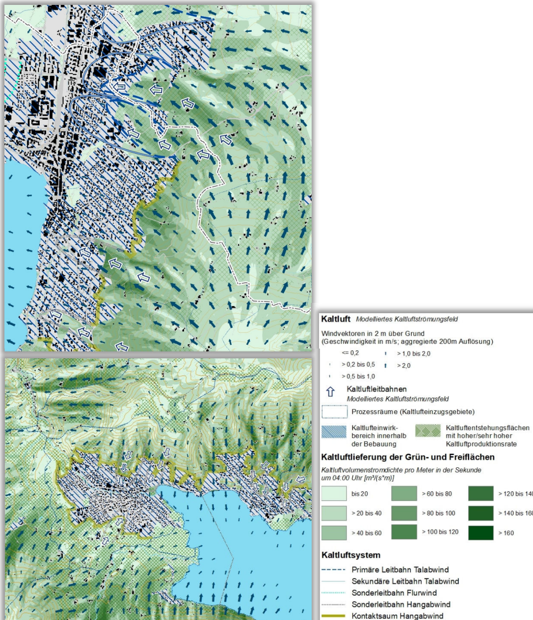
Abb. 5.2: Kaltlufthaushalt in der Nacht in der Stadt Zug (oben) und im Raum Unter-/Oberägeri (unten)
