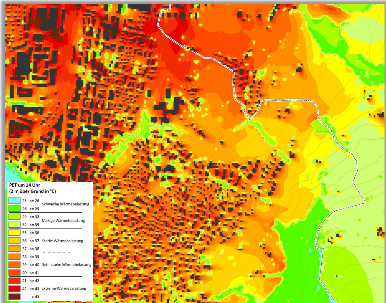
Abb. 4.3: PET in der Stadt Zug zum Zeitpunkt 14 Uhr mittags (2m ü. Grund)
