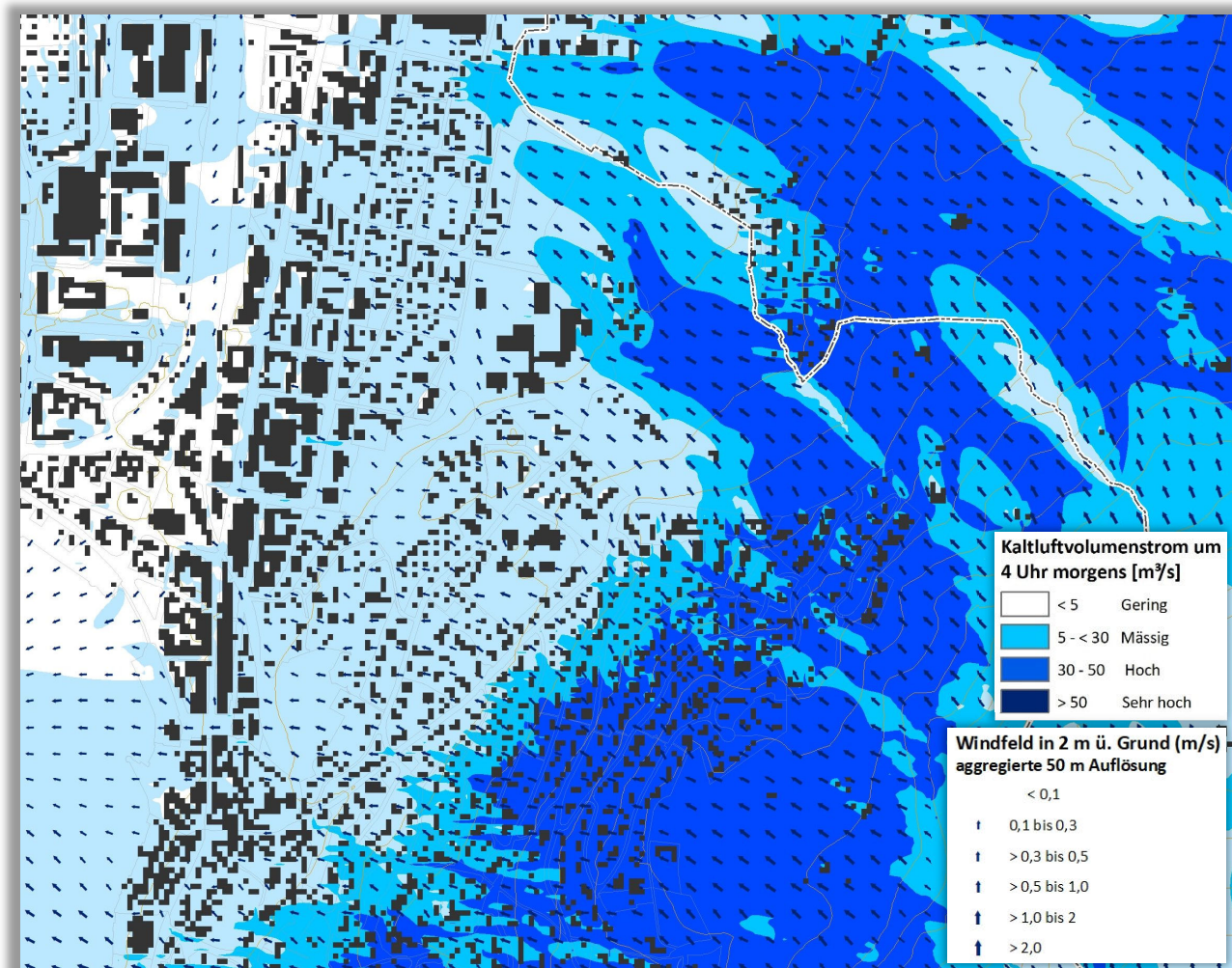
Abb. 4.9: Kaltluftvolumenstrom und bodennahes Windfeld zum Zeitpunkt 4 Uhr morgens in der Stadt Zug (2m ü. Grund)
