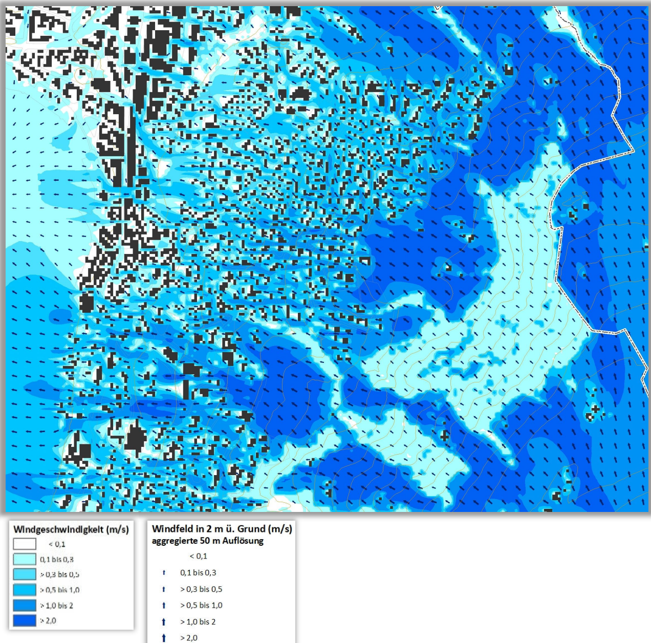
Abb. 4.6: Bodennahes Windfeld zum Zeitpunkt 4 Uhr morgens in der Stadt Zug (2m ü. Grund)
