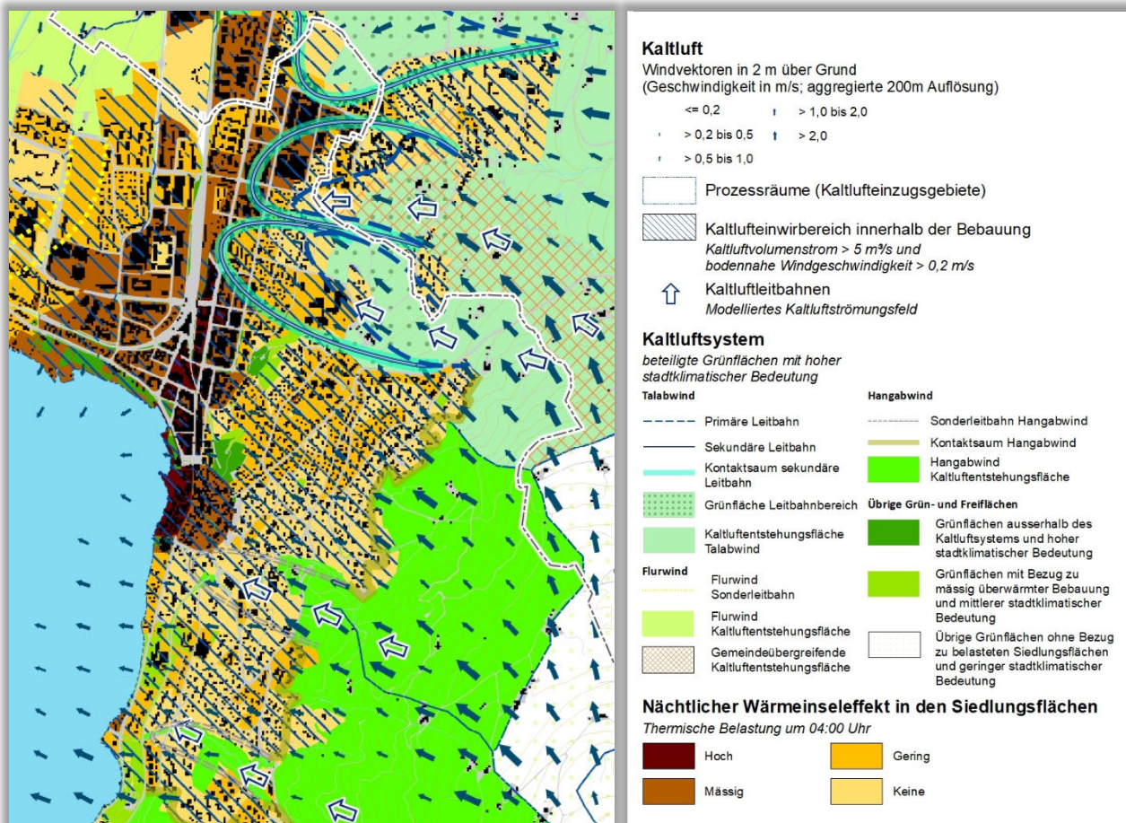
Abb. 6.1: Planungshinweiskarte Nachtsituation in der Stadt Zug
