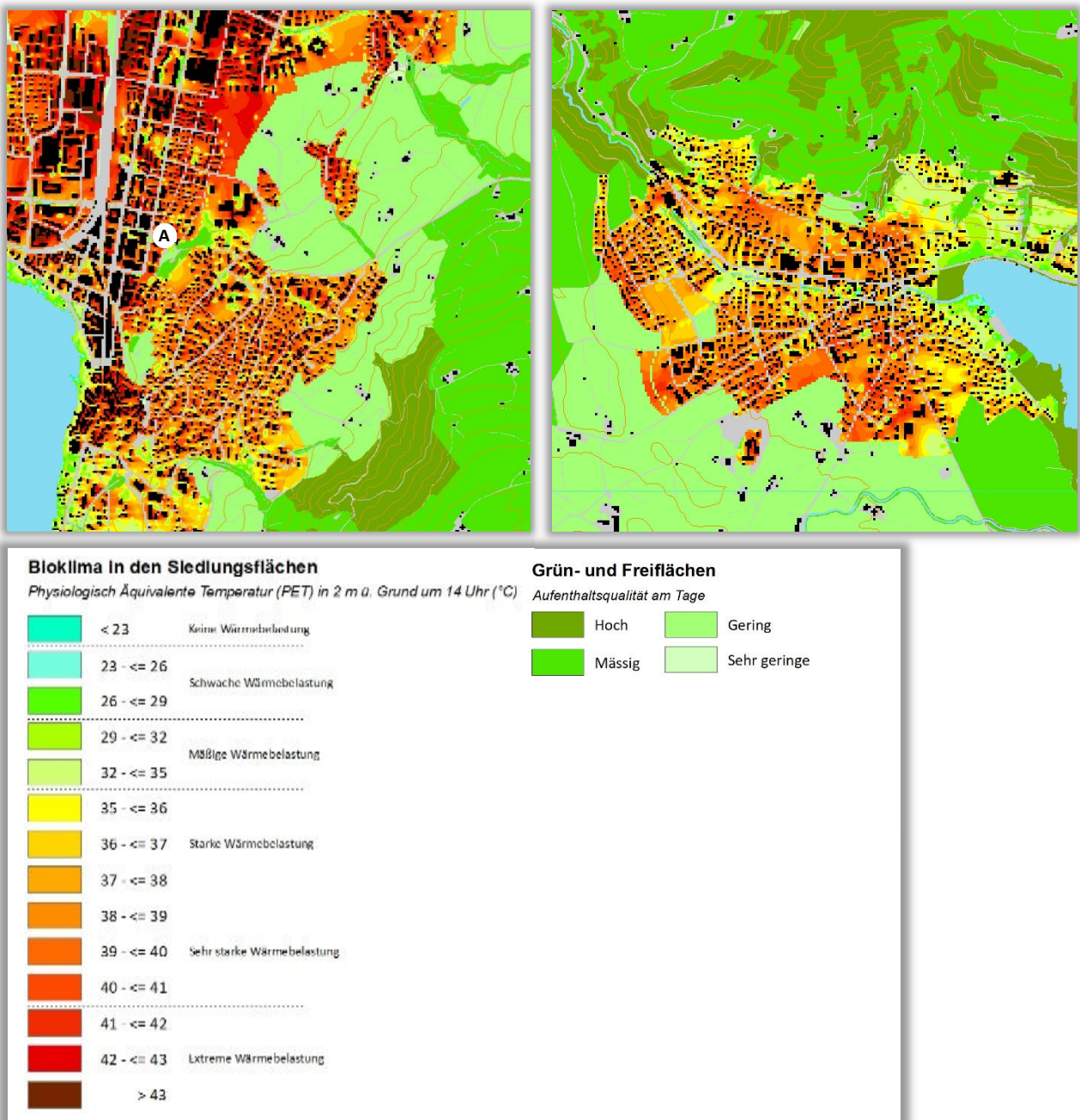
Abb. 6.2: Planungshinweiskarte Tagsituation in der Stadt Zug (links) und Unterägeri (rechts)
