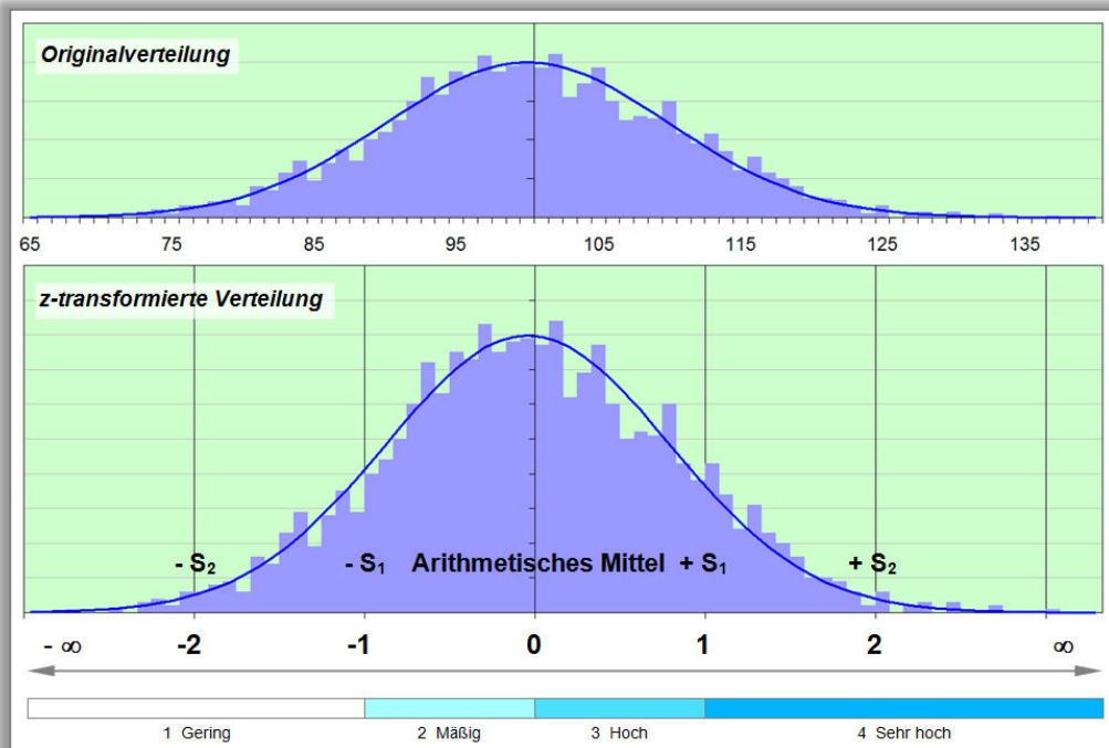
Abb. 4.8: Veranschaulichung der Standardisierung zur vergleichenden Bewertung von Parametern
