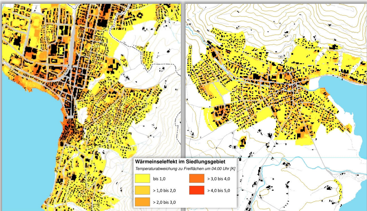
Abb. 5.1: Nächtlicher Wärmeinseleffekt im Siedlungsgebiet (Kernstadt Zug links, Unterägeri rechts)
