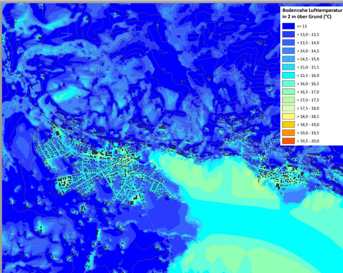
Abb. 4.2: Temperaturfeld im Bereich in Unterägeri und Oberägeri zum Zeitpunkt 4 Uhr morgens (2m ü. Grund)
